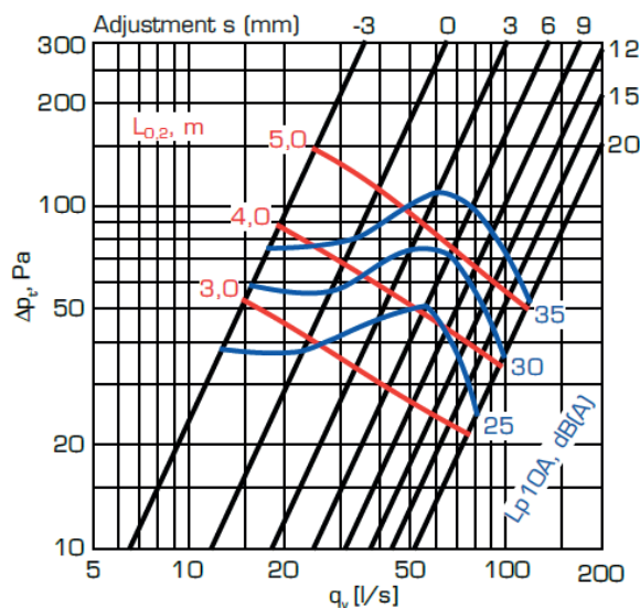
CLU ø200 - Luftstrøm/tryktab/lydniveau
