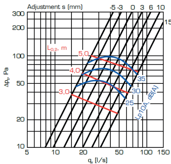
CLU ø200 - Luftstrøm/tryktab/lydniveau
