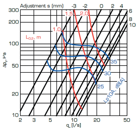
ø100 - Luftfløde / trykfall / ljudnivå
