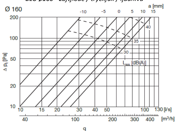
BLU \varnothing 160 - Luftflöde / tryckfall / ljudnivå
