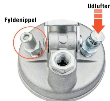
Fedtpresserhoved på GR042700 og GR042720
