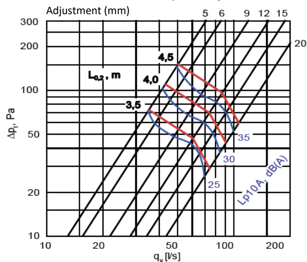
DVI \varnothing 200 - Luftflöde / tryckfall / ljudnivå
