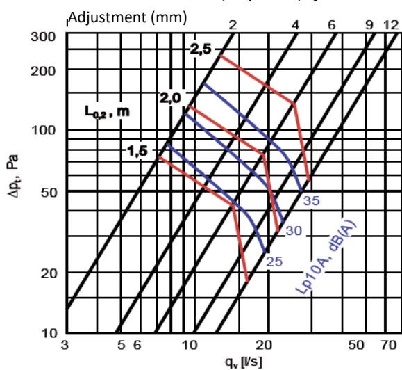
DVI \varnothing 160 - Luftflöde / tryckfall / ljudnivå
