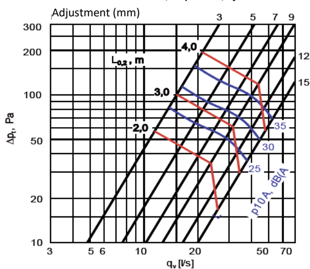
DVI \varnothing 200 - Luftflöde / tryckfall / ljudnivå
