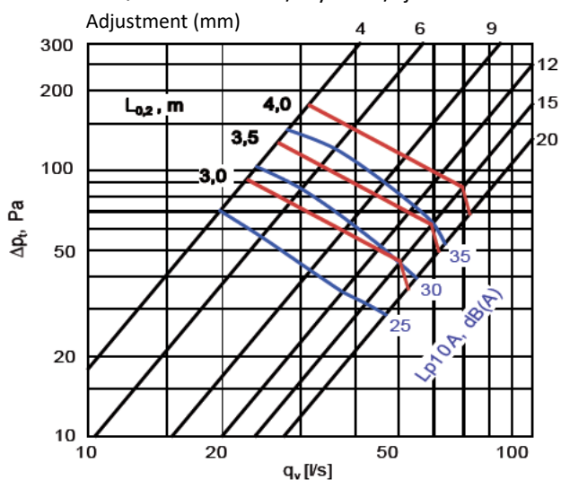
DVI \varnothing 160 - Luftflöde / tryckfall / ljudnivå
